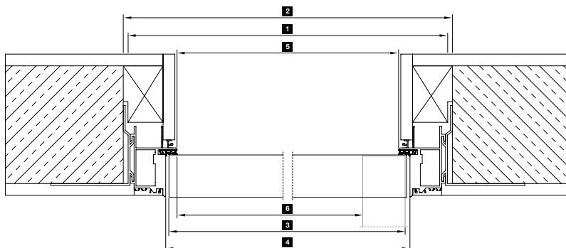
Horizontalni presek krila vrata bez falca
