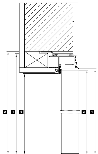
Vertikalni presek krila vrata bez falca
