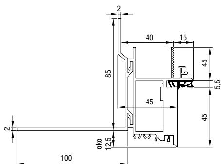
Dimenzije štoka Zeroline
